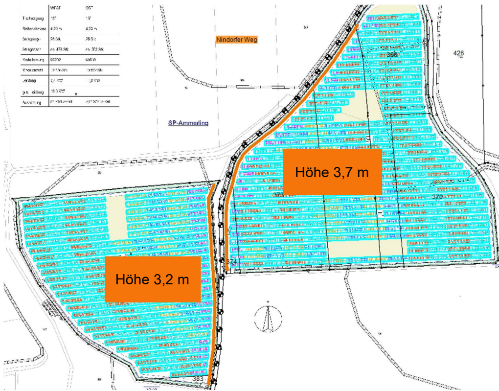
Abbildung 5.1: Lage Blendschutzzaun
