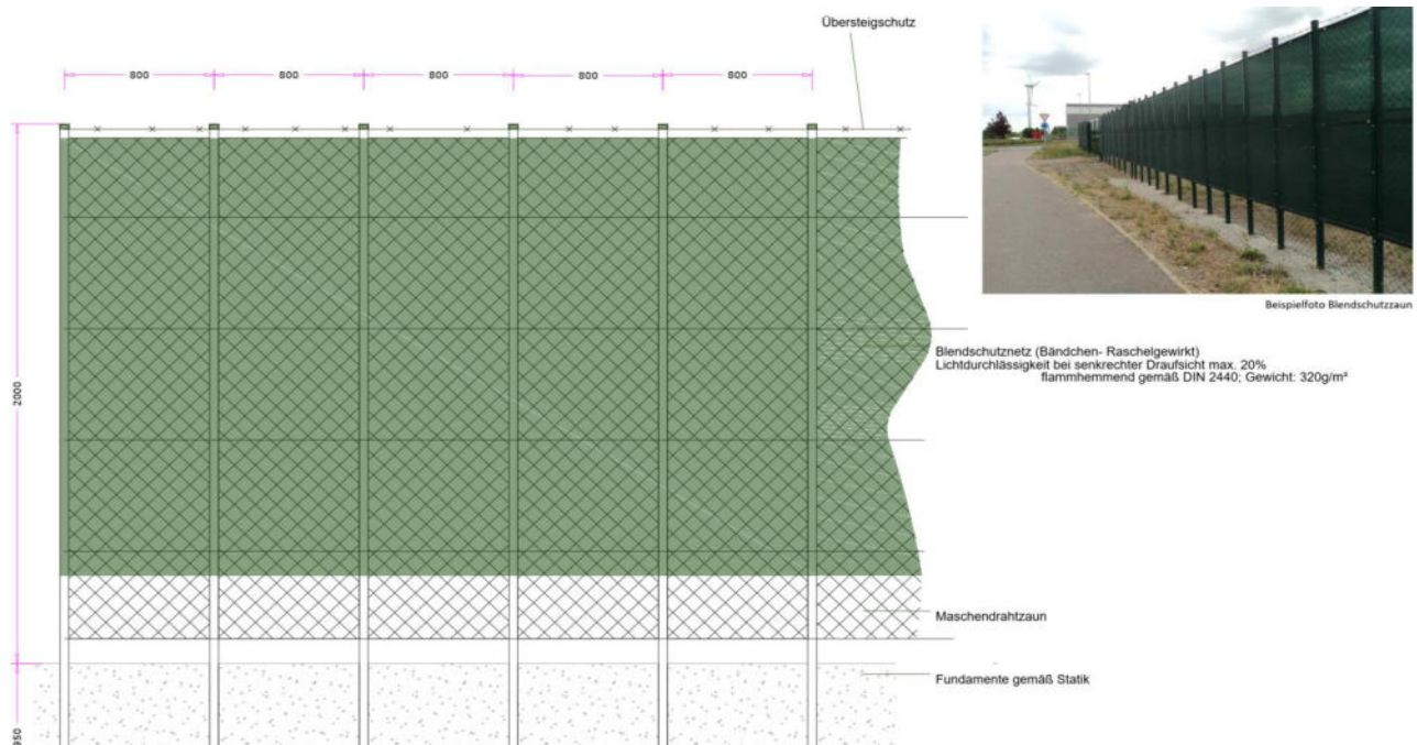
Bild 4.3.4: Beispiel für Sichtschutzmaßnahme (Quelle: Hersteller)
