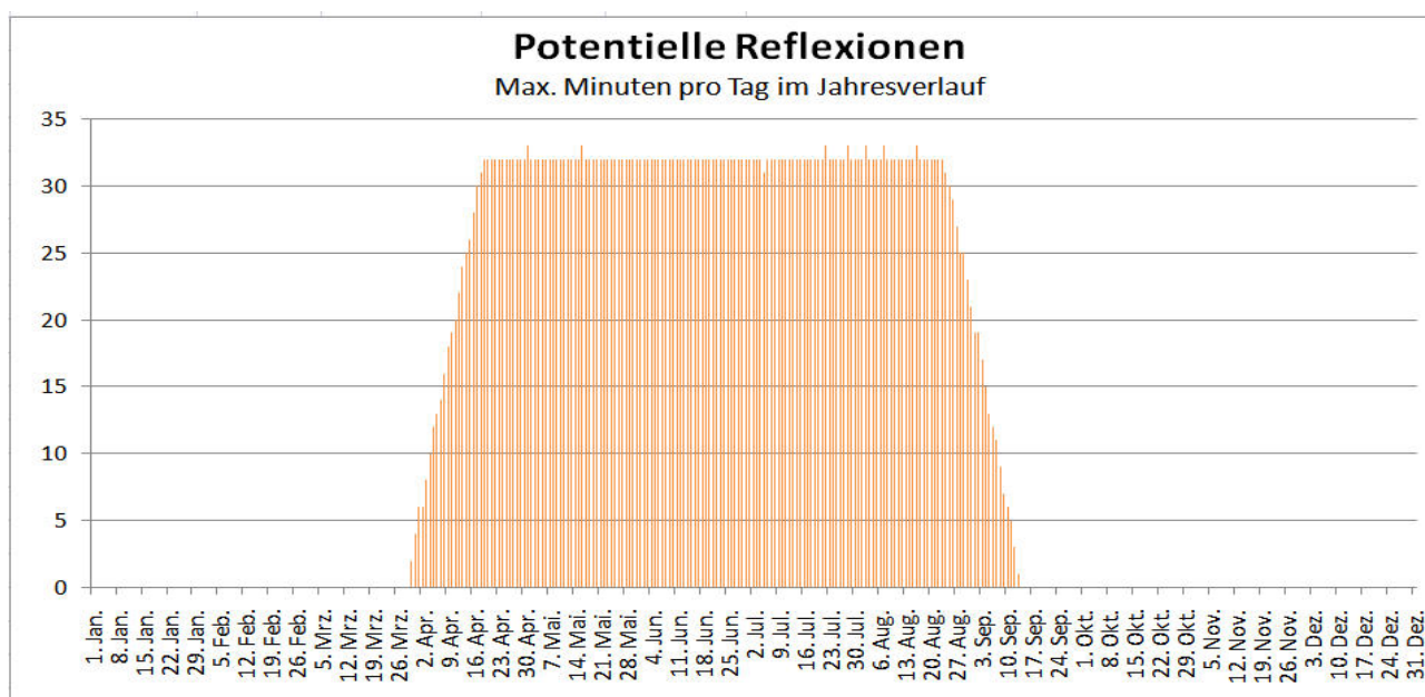
Bild 4.3.2: Reflexionen pro Tag im Jahresverlauf (Quelle: Simulationsergebnisse, aufbereitet)
