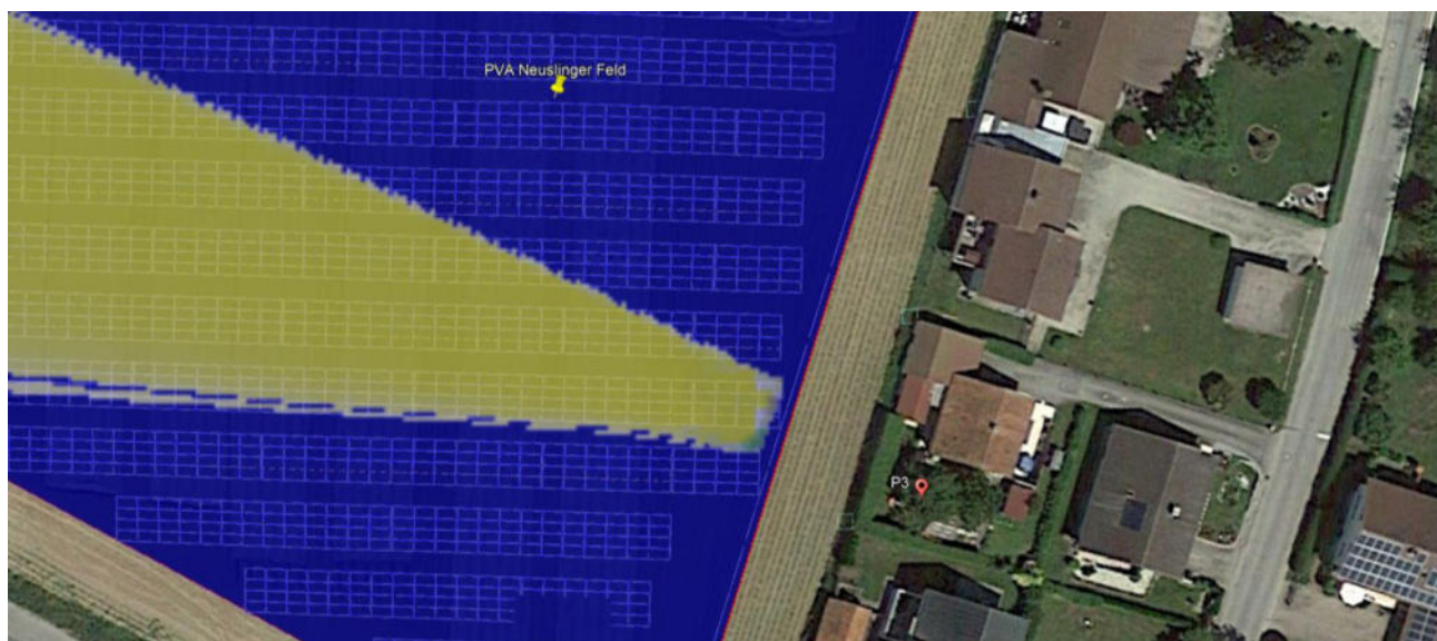
Bild 4.3.1: Simulation am Messpunkt P3 (Quelle: Google Earth/SolPEG)
