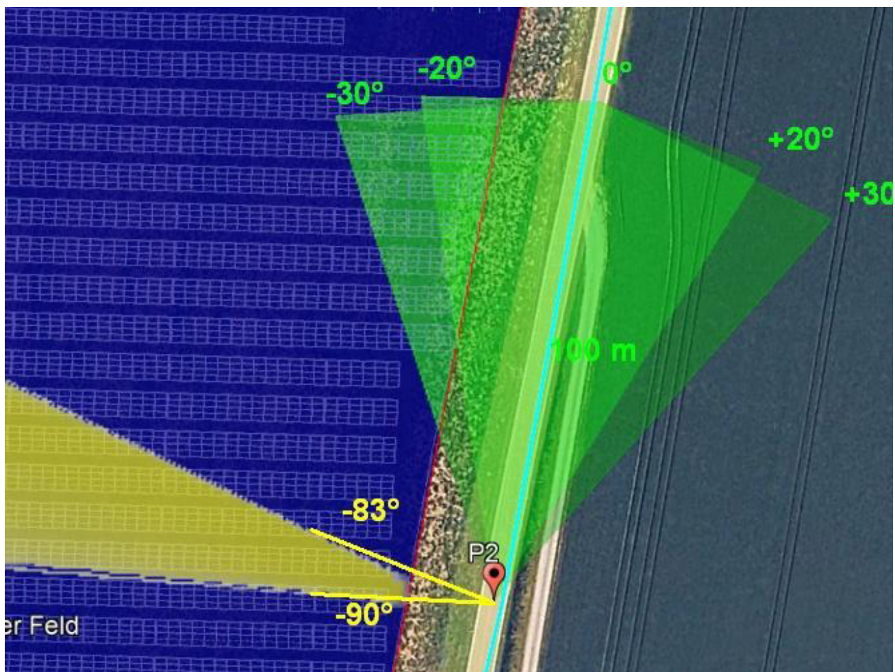
Bild 4.2.1: Simulation am Messpunkt P2 (Quelle: Google Earth/SolPEG)
